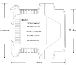
ESCT-RCI-A01/05
