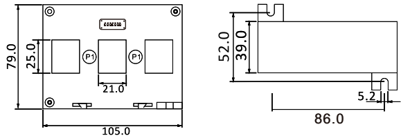
ESCT-SC335
