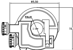
ESCT-P36
