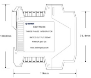
ESCT-RCI-01/03
