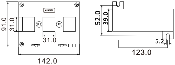
ESCT-SC345
