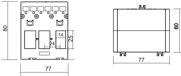
ESCT-C325
