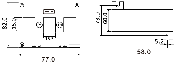
ESCT-SC325
