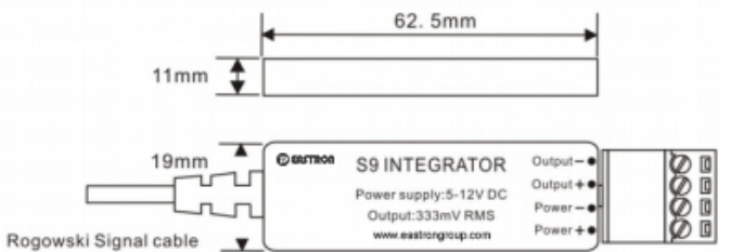
ESCT-RCI-9.1
